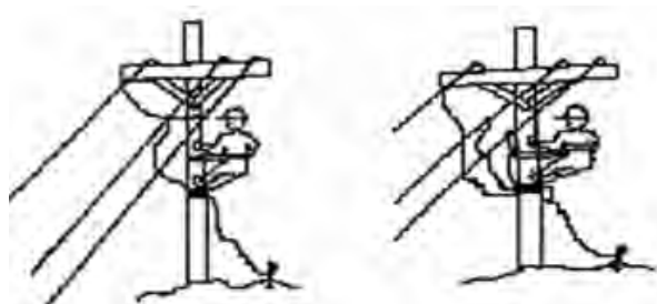
Figura 15.6. Montajes típicos de puestas a tierra temporales
