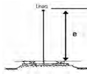
Figura 13.3. Distancia "e" en cruces con ferrocarriles sin electrificar
