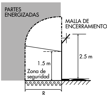
Figura 23.1. Distancias de seguridad para prevenir contactos directos en subestaciones exteriores
