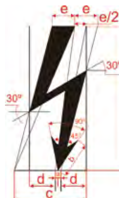
Figura 6.1. Símbolo de riesgo eléctrico
