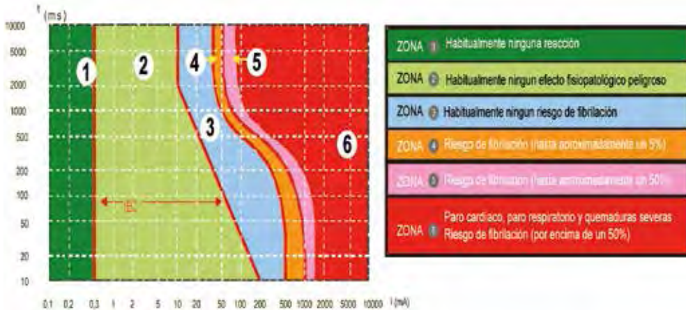
Figura 9.1 Zonas de tiempo/corriente de los efectos de las corrientes alternas de 15 Hz a 100 Hz
