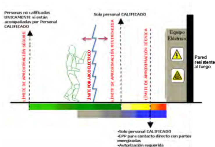
Figura 13.4. Límites de aproximación
