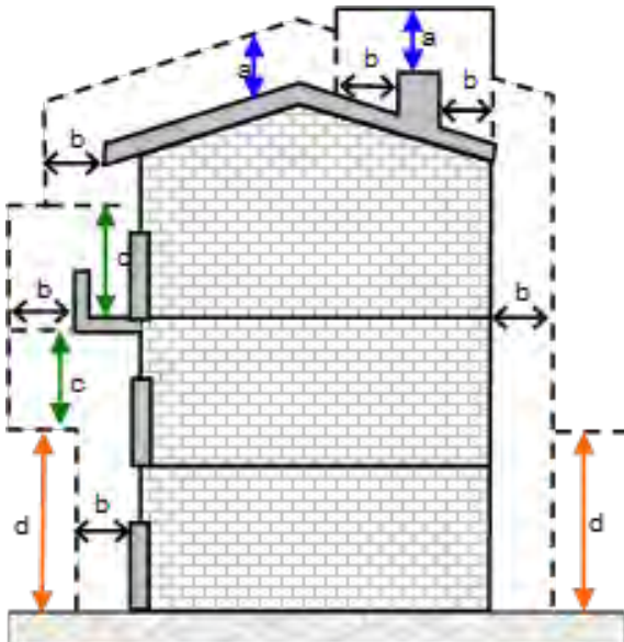
Figura 13.1. Distancias de seguridad en zonas con construcciones
