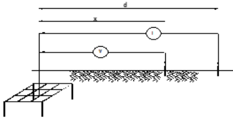
Figura 15.5. Esquema de medición de resistencia de puesta a tierra
