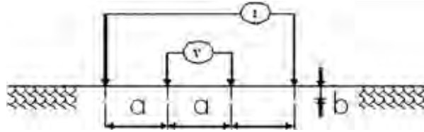
Figura 15.4. Esquema de medición de resistividad aparente
