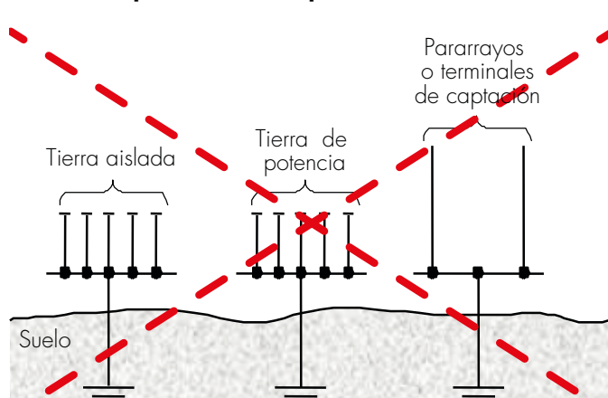
Figura 15.3. Una sola puesta a tierra para todas las necesidades
