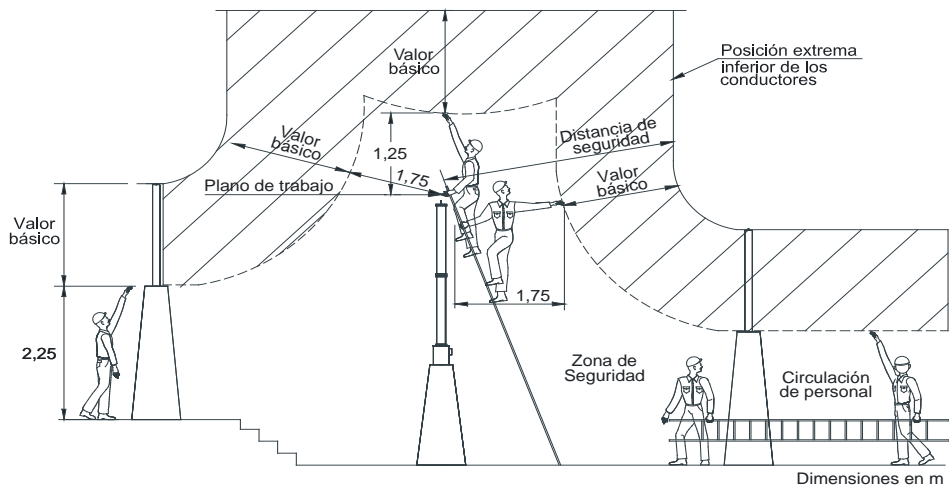
Figura 23.3. Zonas de seguridad
