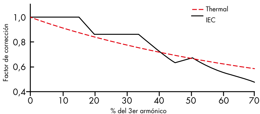
Figura 20.1 Factor de Corrección en función de la proporción de armónicos
