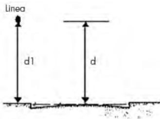
Figura 13.2. Distancias "d" y "d1" en cruce y recorridos de vías
